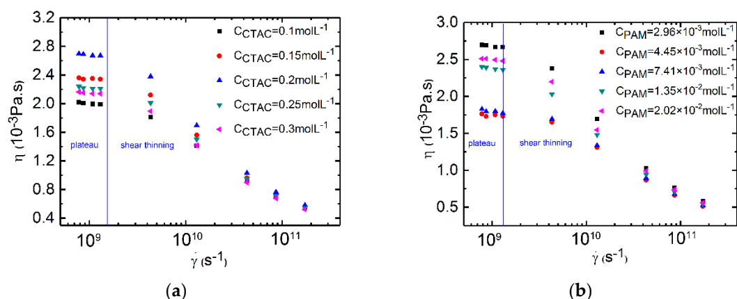
Figure 2. (a) Simulation of shear viscosity versus shear rates for the PAM based solutions. C_{PAM} = 2.96 \times 10^{-3} mol·L -1 , Counter ion salt: NaSal, R = 0.8 , T = 300 K. Black square: C_{CTAC} = 0.1 mol·L -1 . Red circle: C_{CTAC} = 0.15 mol·L -1 . Blue triangle: C_{CTAC} = 0.2 mol·L -1 . Dark cyan triangle: C_{CTAC} = 0.25 mol·L -1 . Magenta triangle: C_{CTAC} = 0.3 mol·L -1 . (b) Simulation of shear viscosity versus shear rates for CTAC based solutions. C_{CTAC} = 0.2 mol·L -1 , counter ion salt: NaSal, R = 0.8 , T = 300 K. Black square: C_{PAM} = 2.96 \times 10^{-3} mol·L -1 . Red circle: C_{PAM} = 4.45 \times 10^{-3} mol·L -1 . Blue triangle: C_{PAM} = 7.41 \times 10^{-3} mol·L -1 . Dark cyan triangle: C_{PAM} = 1.35 \times 10^{-2} mol·L -1 . Magenta triangle: C_{PAM} = 2.02 \times 10^{-2} mol·L -1 .
